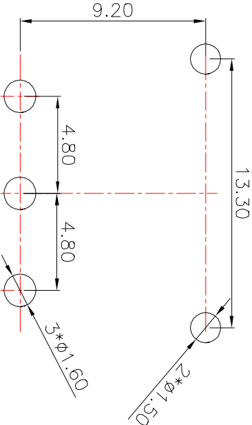
P.C.B layout
