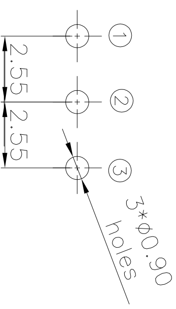
P.C.B layout
