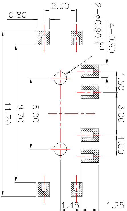
PCB Layout(Pattern side)
