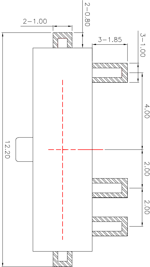
P.C.B layout
