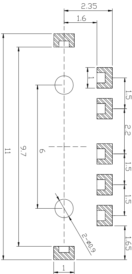
P.C.B layout
