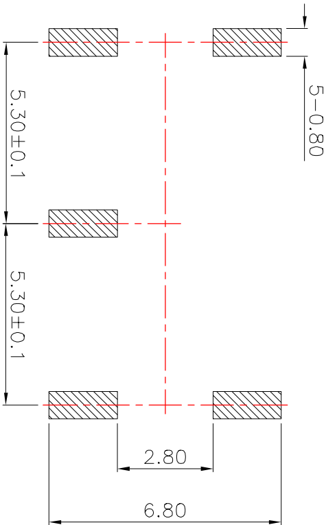
PCB Layout(Pattern side)
