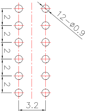
P.C.B layout
