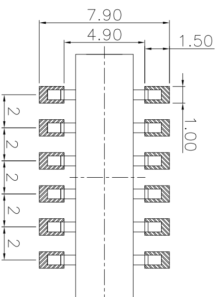
P.C.B layout
