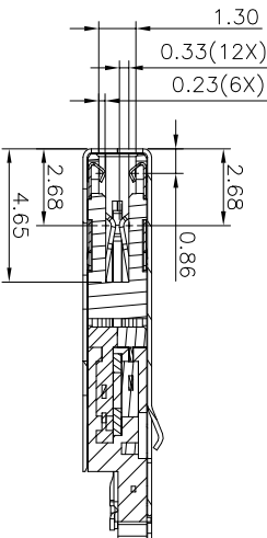
SECTION:A-A SCALE 1:1
