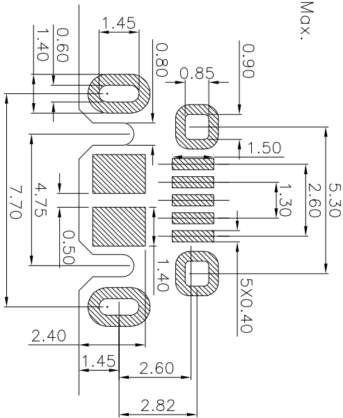
PCB LAYOUT PCB图仅供参考
