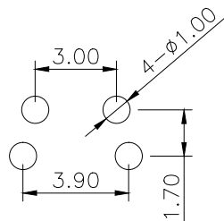
PCB Layout(Pattern side)
