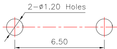
PCB Layout(Pattern Side)
