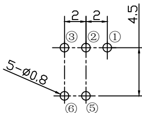
P.C.B 设计参考尺寸
