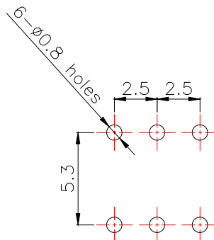
PCB Layout(Pattern Side)
