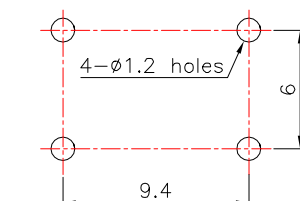
PCB Layout(Pattern Side)
