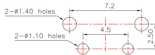
PCB Layout(Pattern side)
