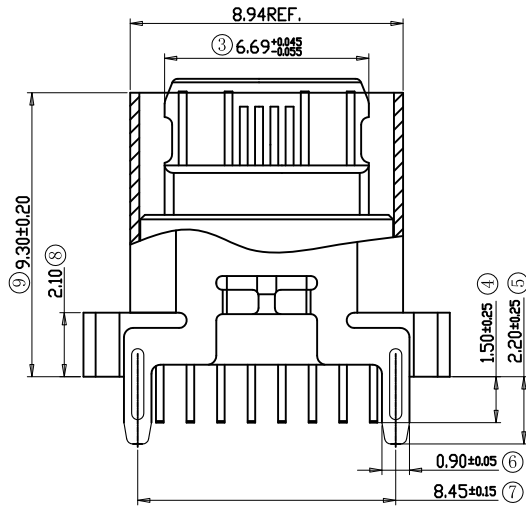
剖视图
