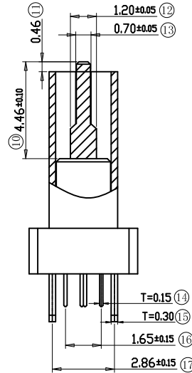
剖视图
