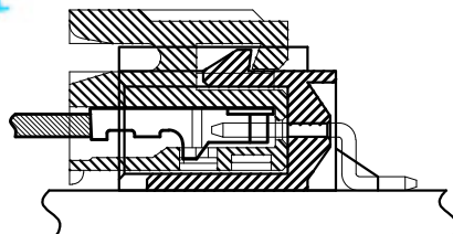
嵌合图面
