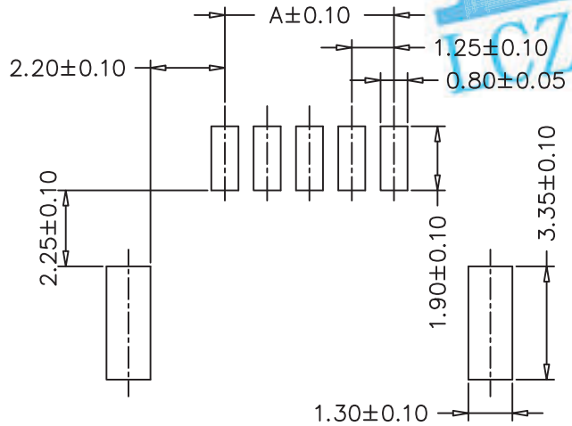
P.C.B. LAYOUT
