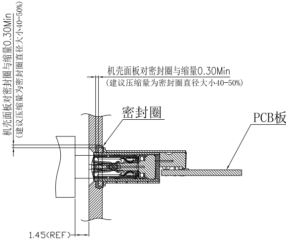
组装面板后公母头对插示意图
