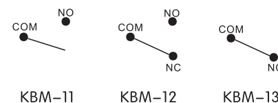
电路图Circuit
