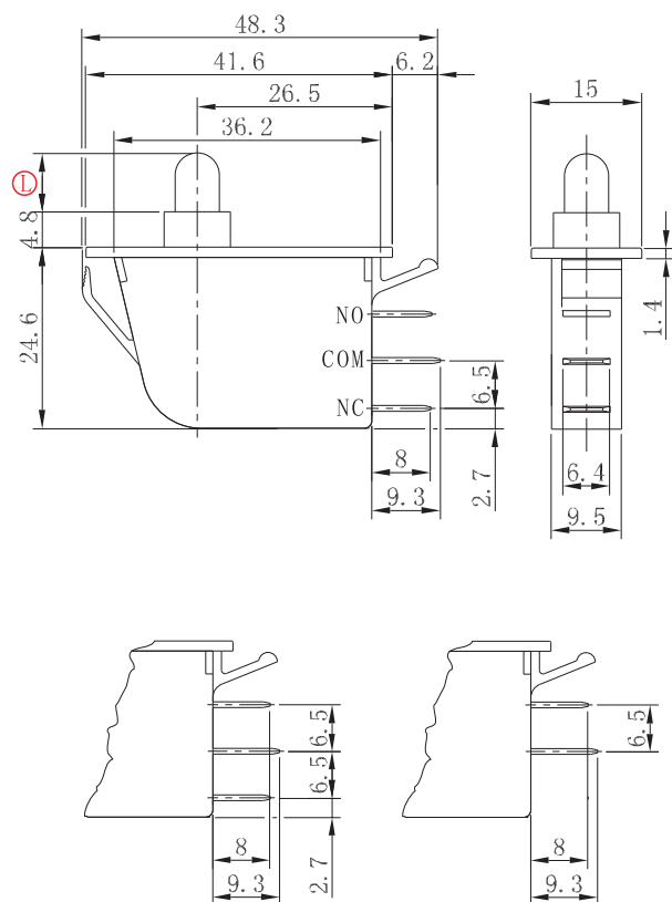
外形尺寸图Overall Dimension(mm)
