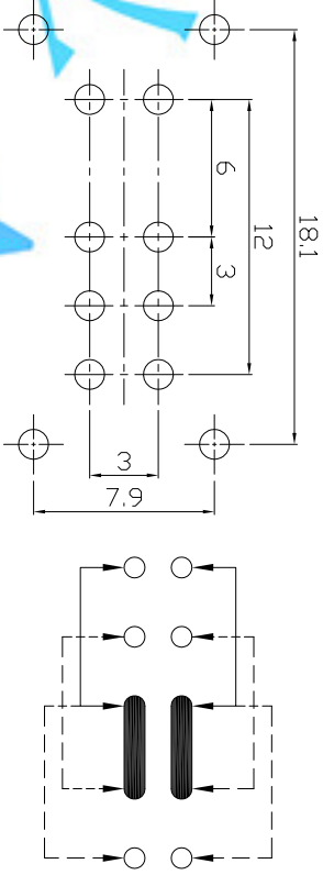
P.C.B LAYOUT
